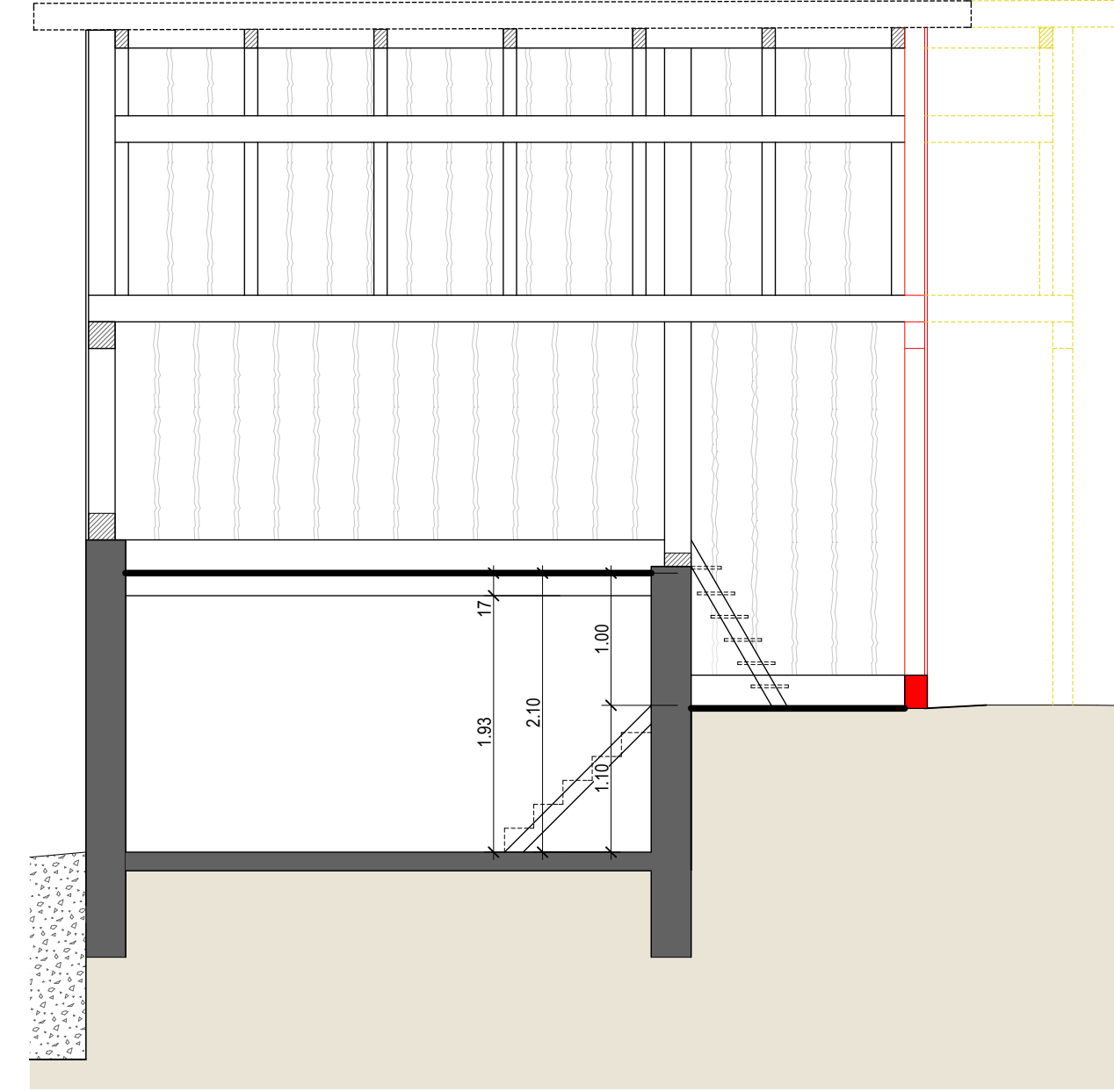
SCHNITT ORT
